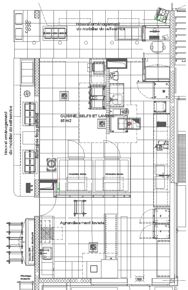
Plan de la cuisine
